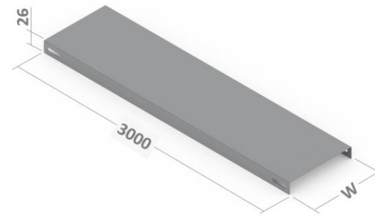
Tampa de encaixe aparafusada Ref. 1010
