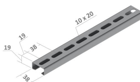
Perfilado perfurado 19x38
