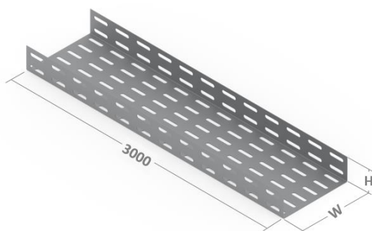
Eletrocalha perfurada na base s/ virolas
