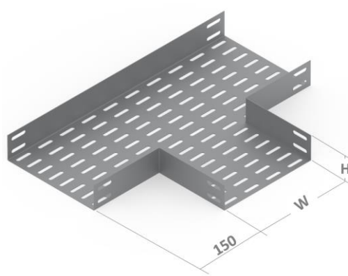
Junção à direita 90° Ref. 1024
