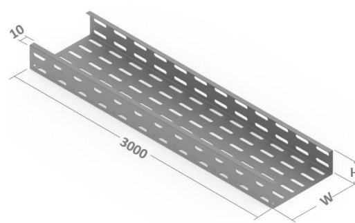
Eletrocalha perfurada na base c/ virolas
