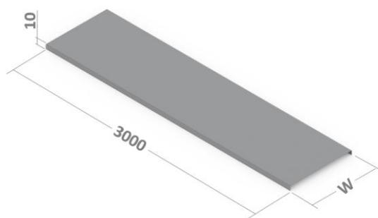
Tampa de encaixe Ref. 1009
