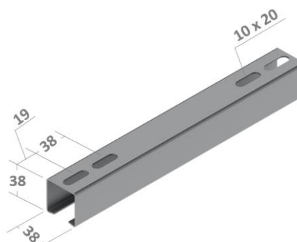
Perfilado perfurado nos extremos 38x38
