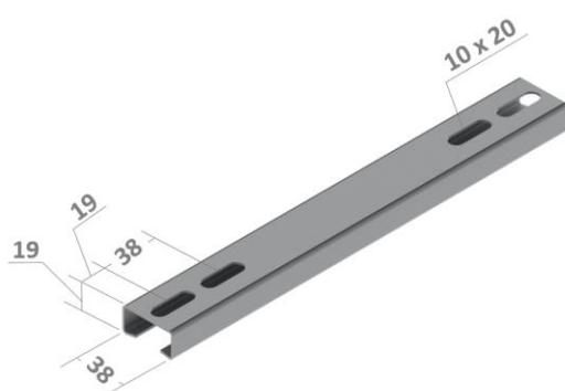
Perfilado liso 38x38 Ref. 2007
