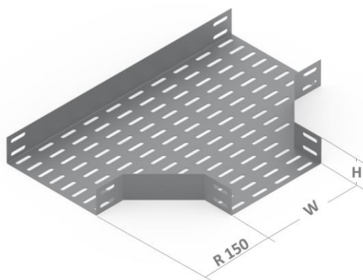
Junção à esquerda 90° Ref. 1023
