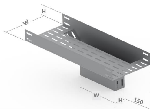
Tê vertical derivação Ref. 1031
