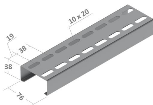
Perfilado perfurado 38x76
