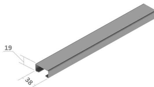
Tampas de encaixe * Comprimento 3000 mm
