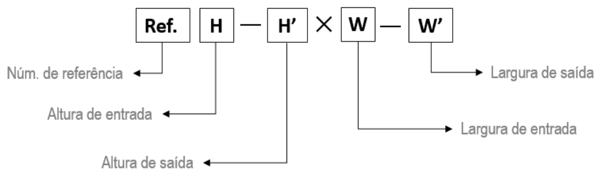
Redução concêntrica Ref. 1036
